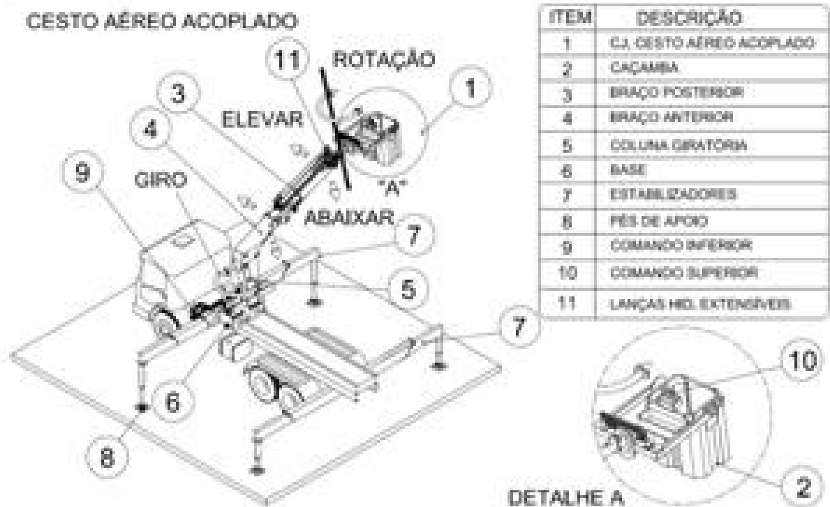
FIGURA 1: EXEMPLO DE ARRANJO COM CESTO ACOPLADO
