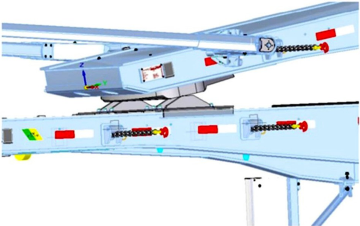
Figura 3: Amarração da carga na região posterior por meio de cintas e catracas
