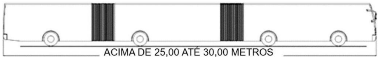
Figura 2 - Veículo biarticulado
